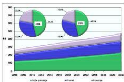
Slika 5-2 Održivi scenarij neposredne potrošnje energije
