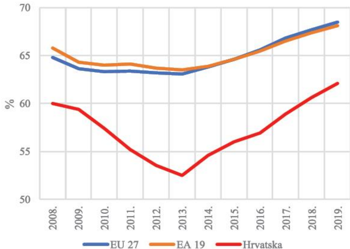
Slika 12. – Stopa zaposlenosti, %
