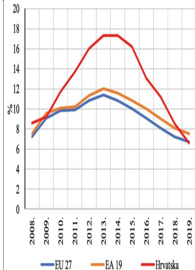
Slika 13. – Stopa nezaposlenosti, %
